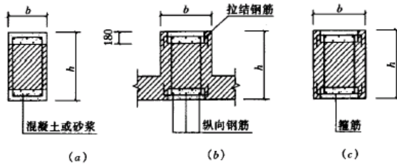
图 8.2.1 组合砖砌体构件截面
