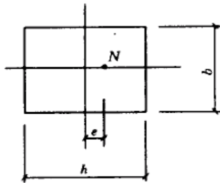
图 D.0.1 单向偏心受压
