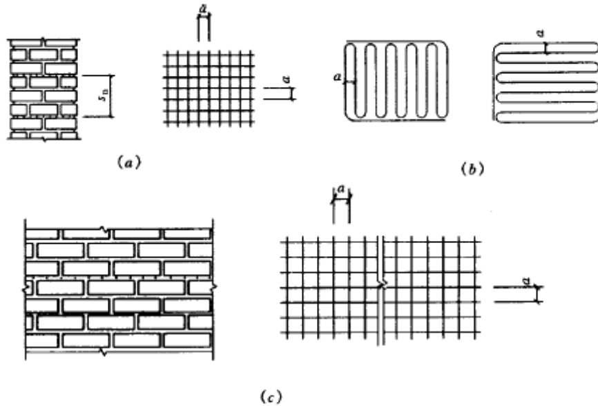
图 8.1.2 网状配筋砌体
