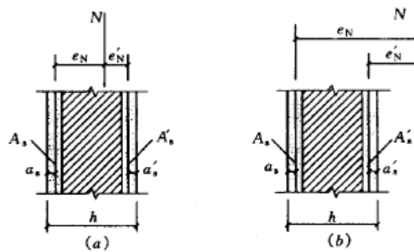
图 8.2.4 组合砖砌体偏心受压构件
