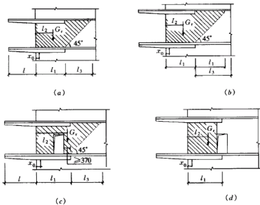
图 7.4.3 挑梁的抗倾覆荷载
