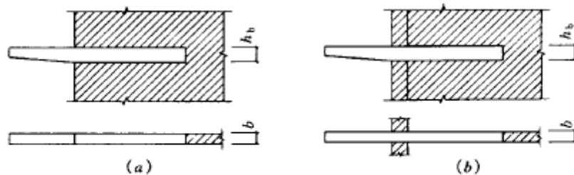
图 7.4.4 挑梁下砌体局部受压
