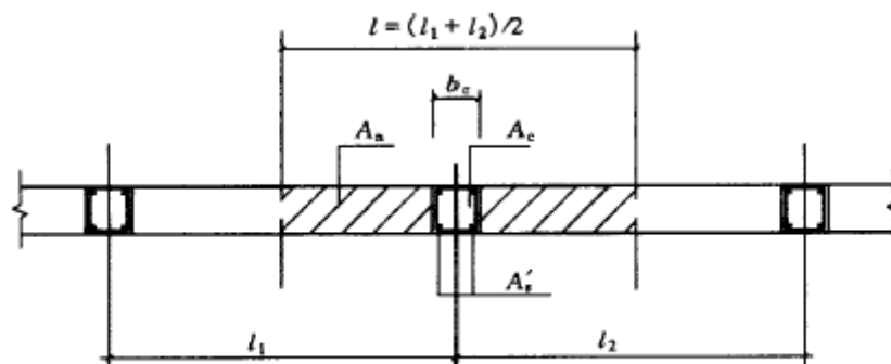
图 8.2.7 砖砌体和构造柱组合墙截面
