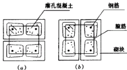
图 9.4.14 配筋砌块砌体柱截面示意
