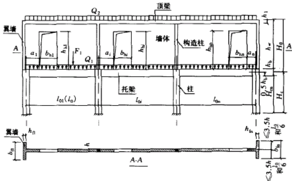
图 7.3.3 墙梁的计算简图
