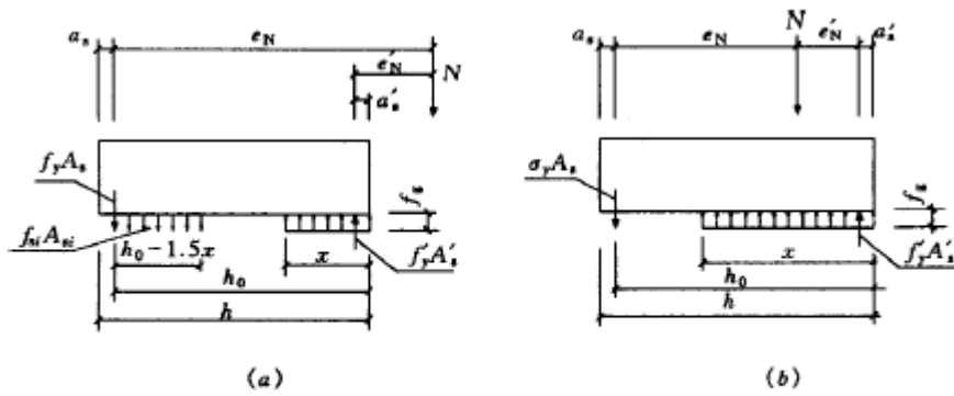
图 9.2.4 矩形截面偏心受压正截面承载力计算简图 (a) 大偏心受压; (b) 小偏心受压
