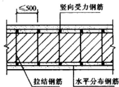
图 8.2.6 混凝土或砂浆 面层组合墙
