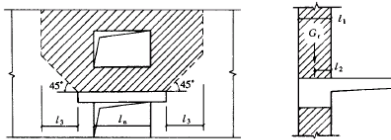
图 7.4.7 雨篷的抗倾覆荷载
