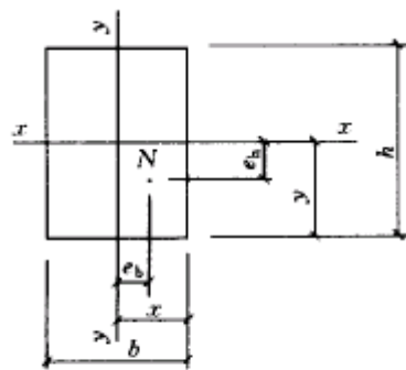
图 D.0.2 双向偏心受压
