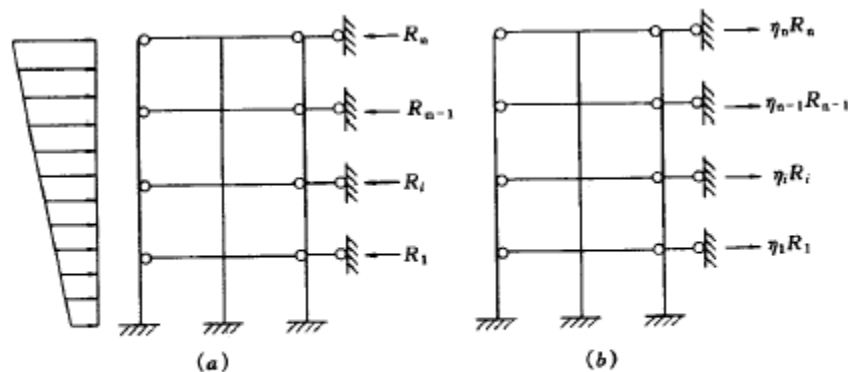
图 C 刚弹性方案房屋的静力计算简图
